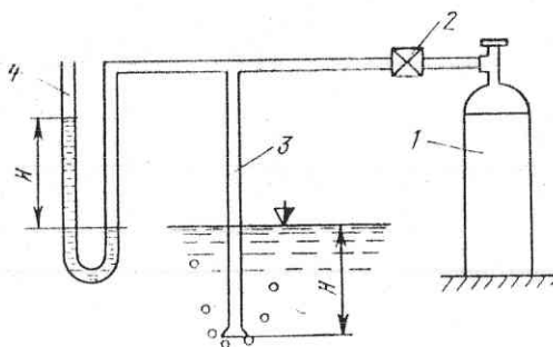
Рис. 5-7. Схема пневмогидравлического способа измерения уровня воды. 1 — баллоны с сжатым воздухом или ресивер; 2 — дроссель; 3 — трубка подачи воздуха под уровень воды; 4 — воздушнo-водяной или пружинный манометр.
