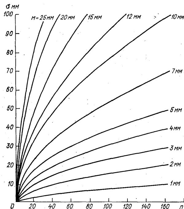
Рис. 20. График для определения числа скважин n , обеспечивающих получение среднего запаса влаги в почвогрунтах на водосборе с ошибкой \sigma_{0,8} (обеспеченность неперевышения 80 %).
