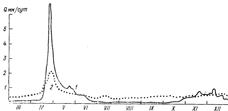
Рис. 17. Гидрографы стока с лесных водосборов Валдайского филиала ГГИ, сложенных различными грунтами, в маловодный 1964 г.
