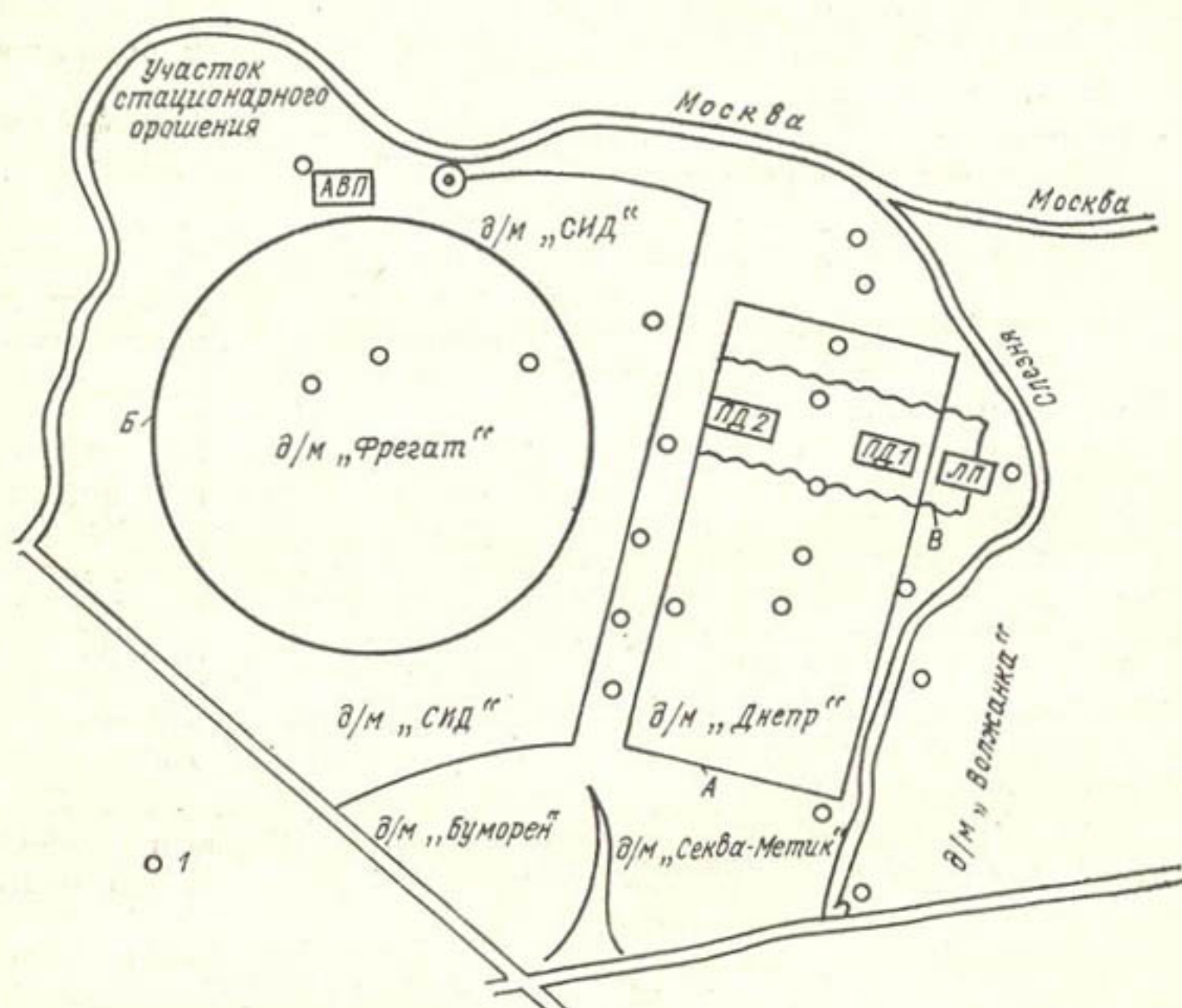
Рис. 4.10. Схема размещения дождевальных машин (д/м), грунтовых скважин (I) и дренажа на мелноративной системе «Горки-2».
