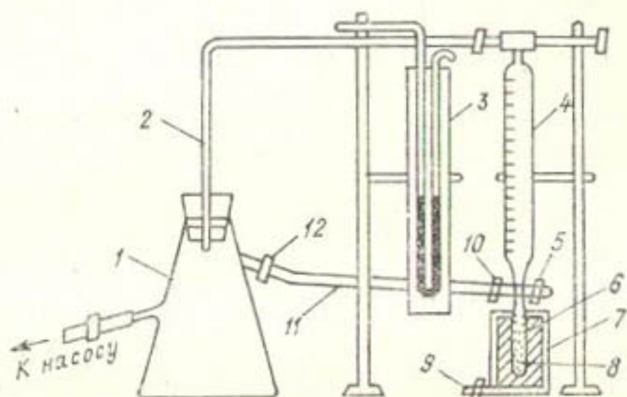
Рис. 2.5. Схема капилляриметрической установки.
