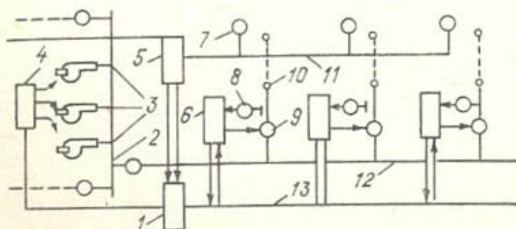
Рис. 6.1. Структурная схема автоматической системы полива сельскохозяйственных культур.
