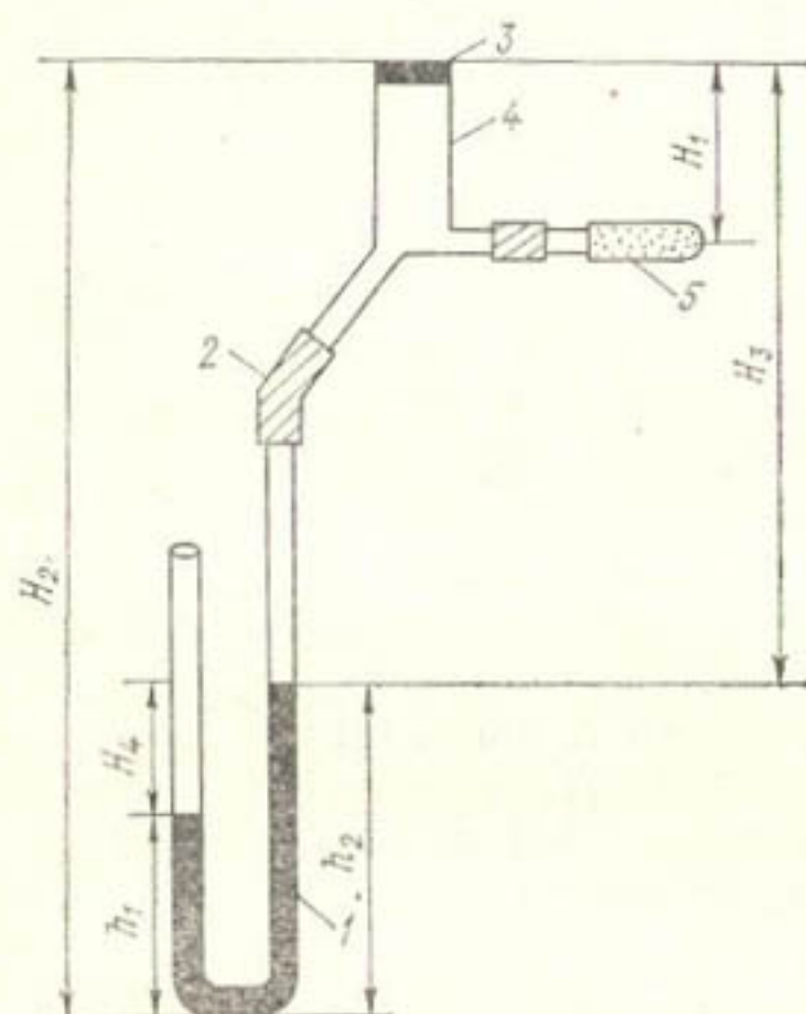
Рис. 2.7. Схема лабораторной модели тензиометра.
