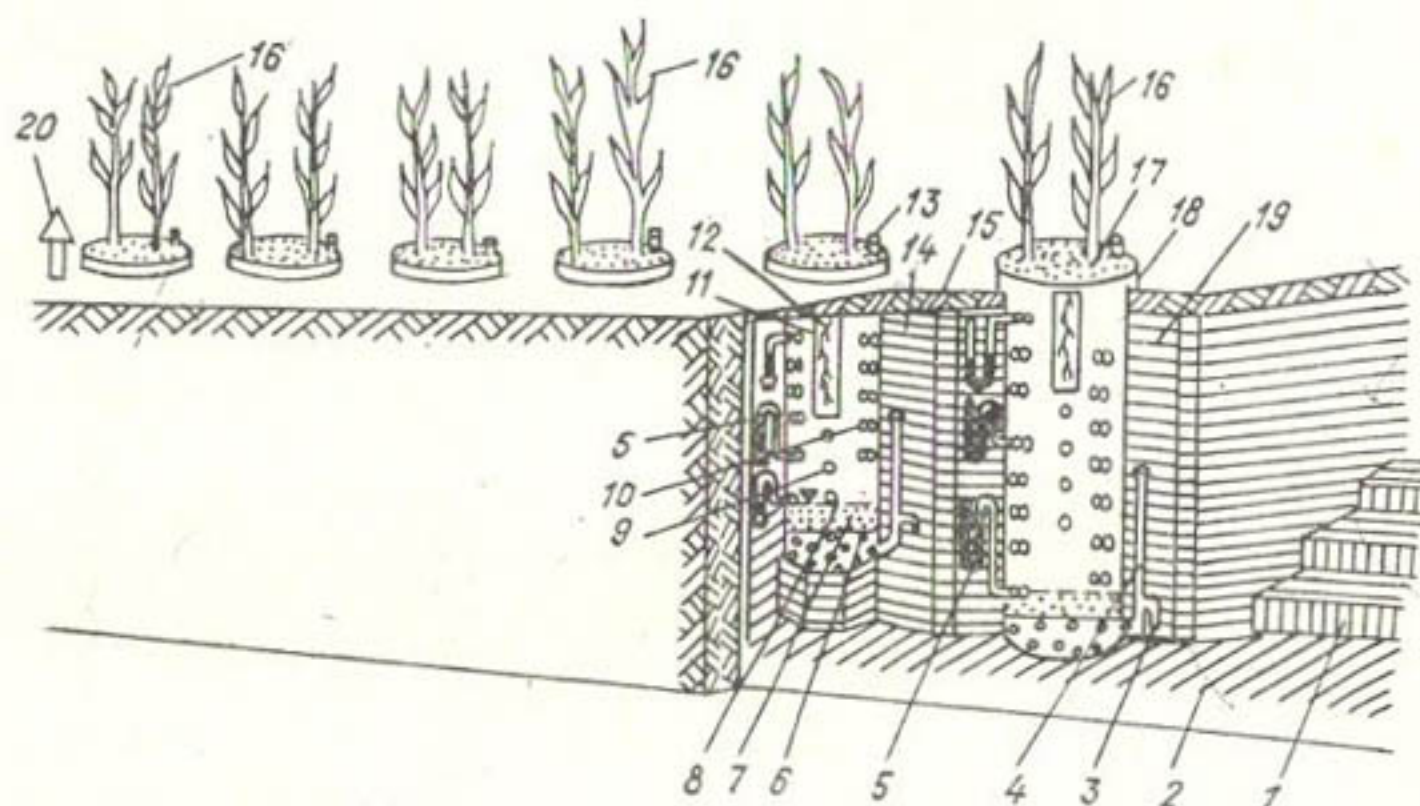
Рис. 4.2. Схема устройства лизиметрического павильона.
