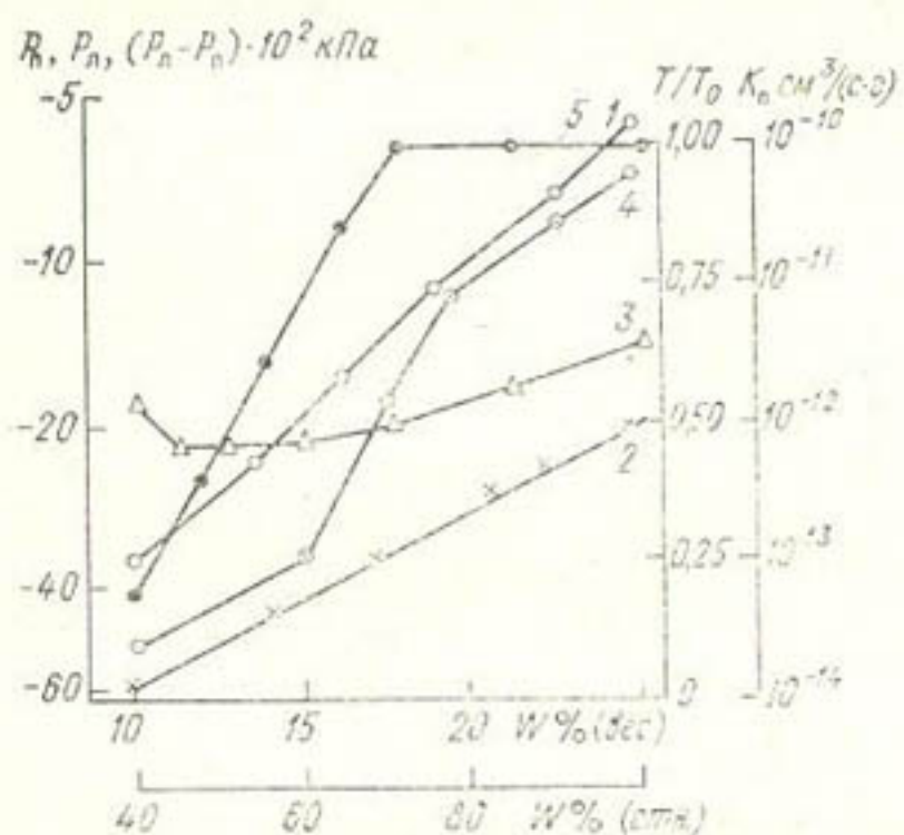
Рис. 5.4. Зависимость потенциала влаги в почве ( P_n ) и листьях проса ( P_l ), перепада потенциала ( P_l - P_n ), коэффициента влагопроводности почвы ( K_n ) и относительной транспирации ( T/T_0 ) от влажности черноземовидной суглинистой почвы.
