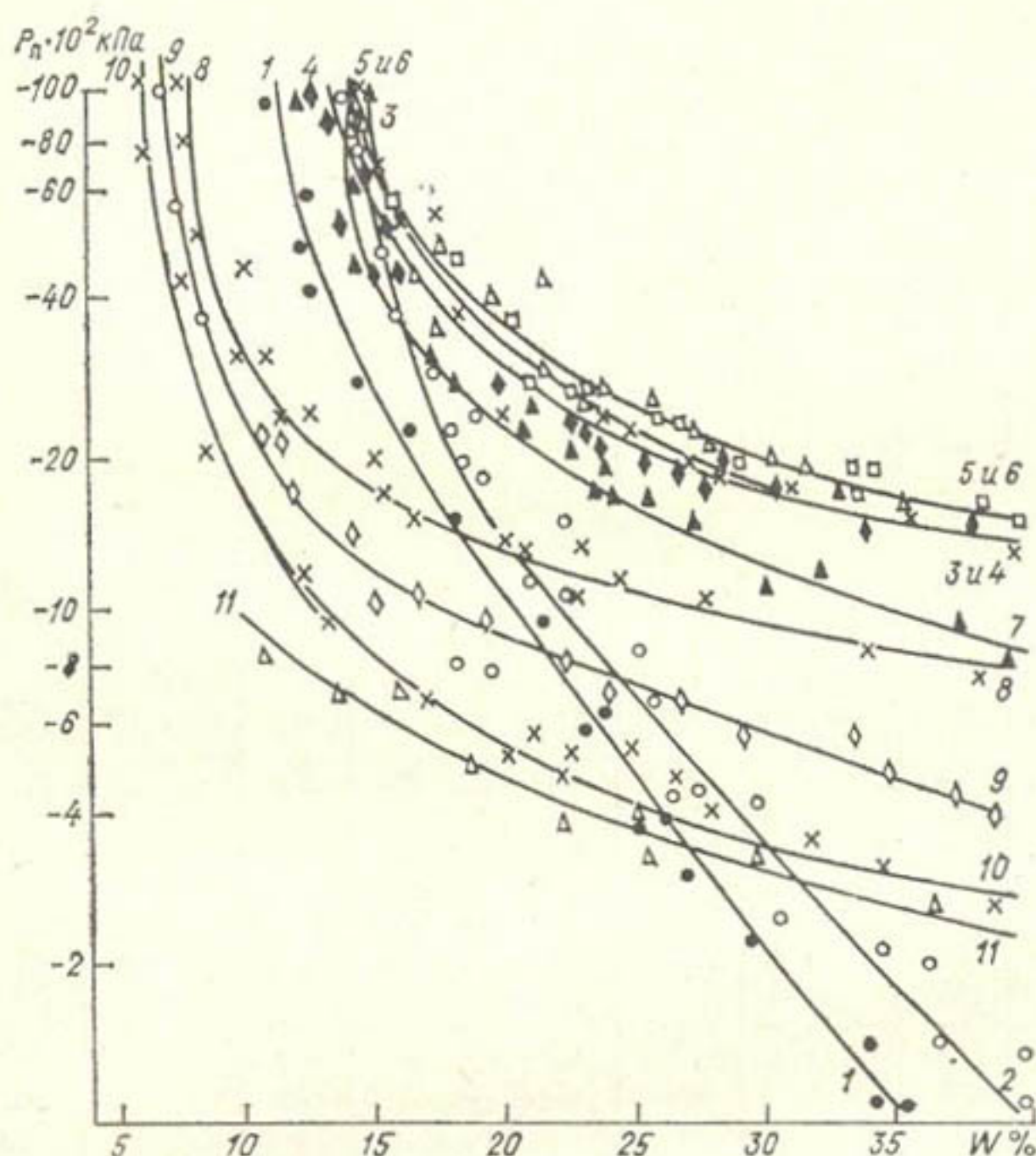
Рис. 3.9. Зависимость полного потенциала почвенной влаги P_n от влажности почвы в солончаковом солонце.
