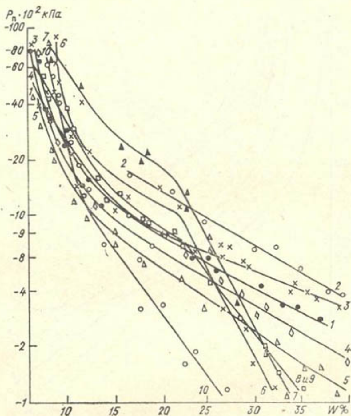
Рис. 3.7. Зависимость полного потенциала почвенной влаги P_n от влажности в темноцветной почве.
