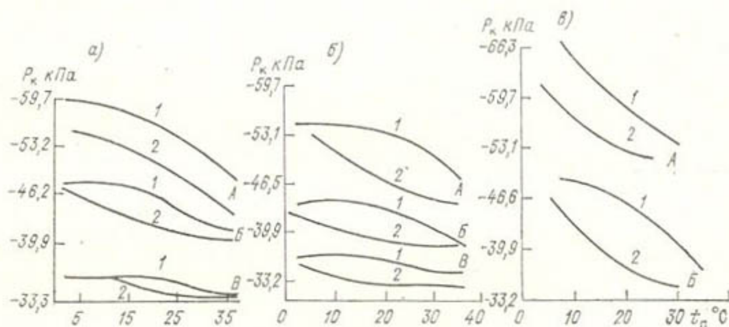
Рис. 3.13. Зависимость потенциала почвенной влаги P_k от температуры t_n в аллювиальной луговой суглинистой (а), дерново-подзолистой песчаной (б) и иловато-торфяной (в) почвах.
