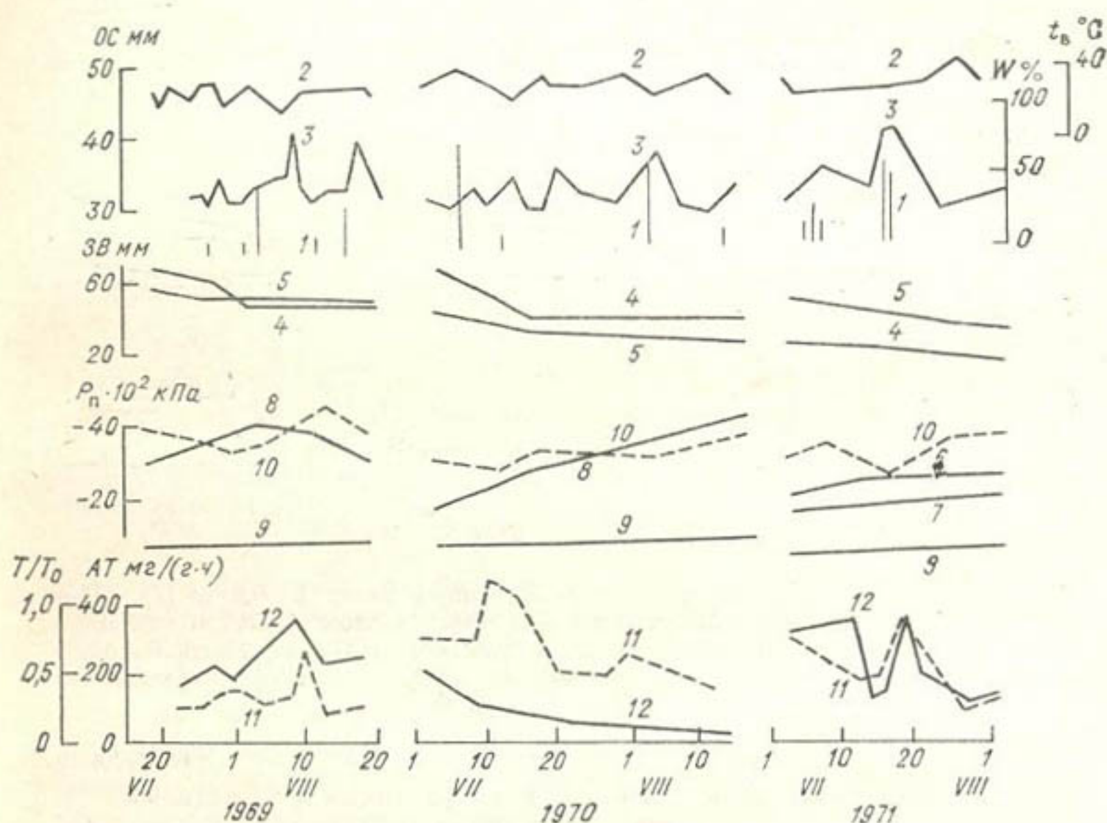
Рис. 5.11. Динамика осадков (1), температуры воздуха (2), относительной влажности воздуха (3) в 13 ч, запасов влаги в слоях почвы 0—100 см (4) и 100—200 см (5), потенциала почвенной влаги в слоях 0—50 см (6), 50—100 см (7), 0—100 см (8) и 100—200 см (9), потенциала влаги в хвое сосны (10), абсолютной транспирации (11) и относительной транспирации (12) в сосновых насаждениях 10-летнего возраста.
