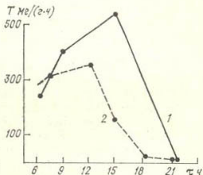
Рис. 5.13. Суточный ход транспирации сосновых насаждений 10-летнего (1) и 40-летнего (2) возраста.
