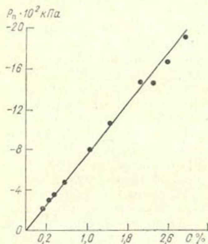
Рис. 3.10. Зависимость потенциала почвенной влаги P_p от содержания водорастворимых солей C .
