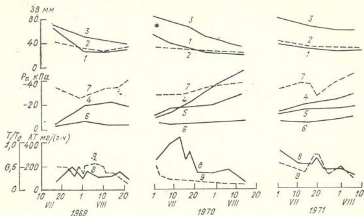
Рис. 5.12. Динамика запасов влаги в почвенных слоях 0—0,5 м (1), 0,5—1,0 (2), 1—2 м (3), потенциала почвенной влаги в слоях 0—0,5 м (4), 0,5—1,0 (5), 1—2 м (6), потенциала влаги в хвое сосны (7), абсолютной транспирации (8) и относительной транспирации (9) в сосновых насаждениях 40-летнего возраста.
