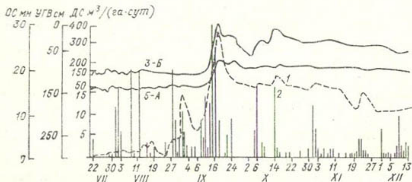
Рис. 4.11. Динамика грунтовых вод, осадков и дренажного стока с июля по декабрь 1981 г.
