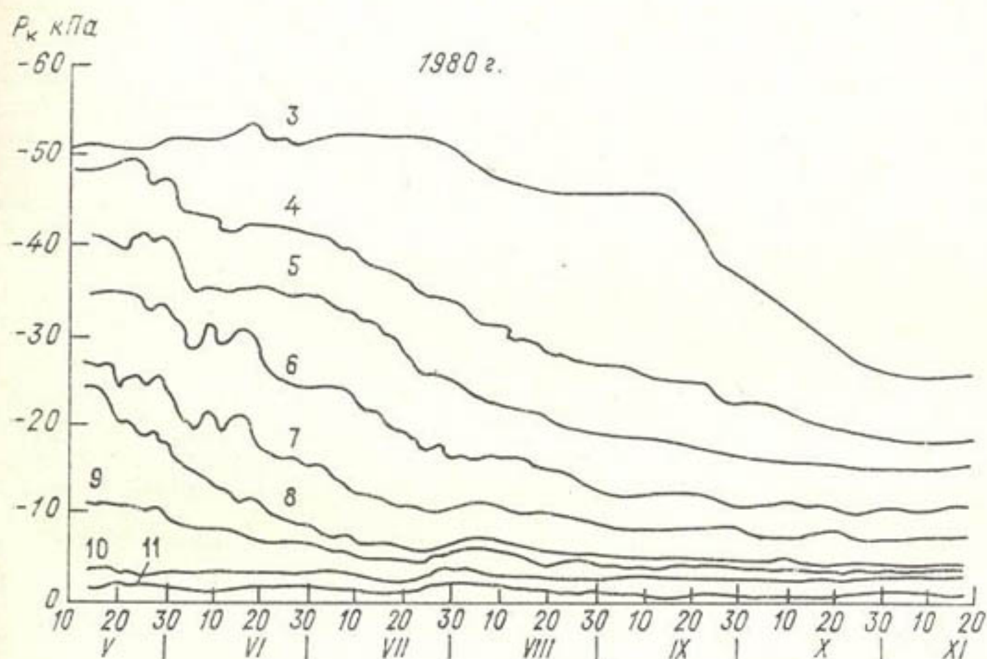
Рис. 4.6. Динамика потенциала почвенной влаги P_k в аллювиальной луговой суглинистой почве ненарушенного сложения.
