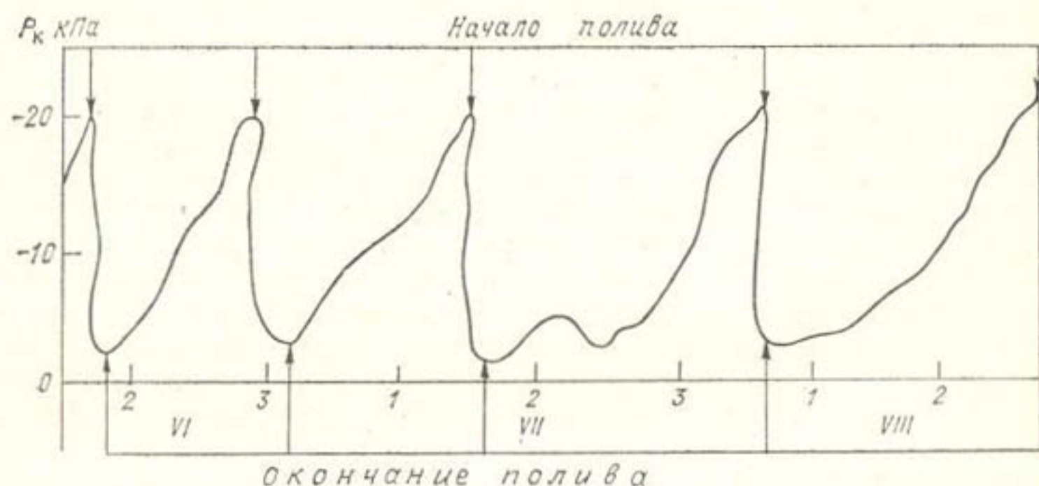
Рис. 6.3. Динамика потенциала влаги в слое 20—25 см аллювиальной дерново-суглинистой почвы в условиях автоматического полива кукурузы (1979 г.).
