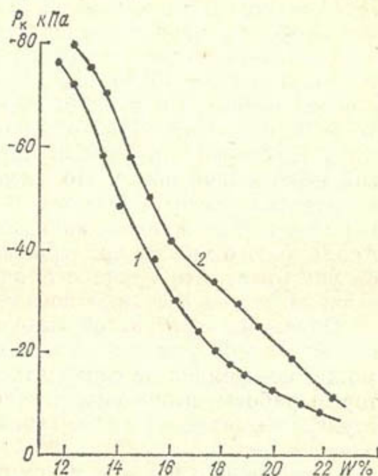
Рис. 3.12. Зависимость капиллярно-сорбционного потенциала влаги P_k от влажности в слое 105—150 см в светло-каштановой почве солонцового комплекса Северного Прикаспия. 1 — данные тензиометров, заправленных дистиллированной водой, 2 — данные тензиометров, заправленных раствором поваренной соли.
