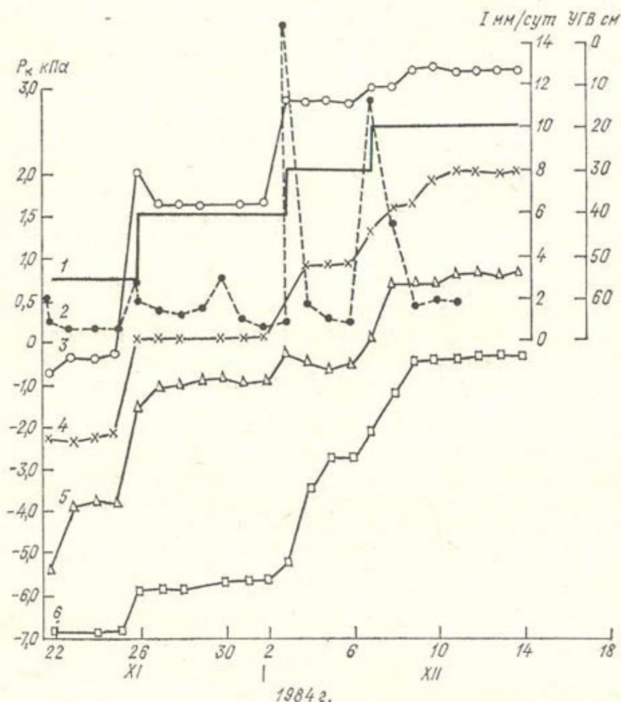
Рис. 4.7. Динамика потенциала влаги P_k , УГВ и интенсивности расхода грунтовых вод I .
