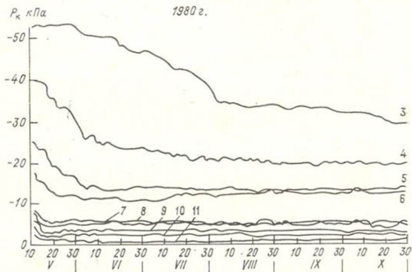
Рис. 4.5. Динамика потенциала почвенной влаги P_k в аллювиальной луговой суглинистой почве нарушенного сложения.
