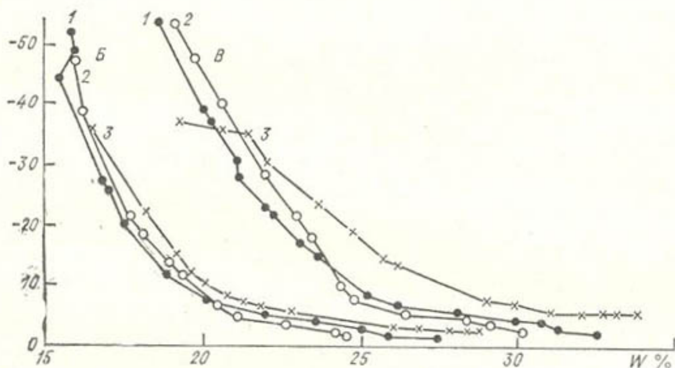
Рис. 3.15. Зависимость потенциала влаги P_k от влажности в слоях 190—200 см (А), 80—90 см (Б) и 40—50 см (В) аллювиальной луговой суглинистой почвы.
