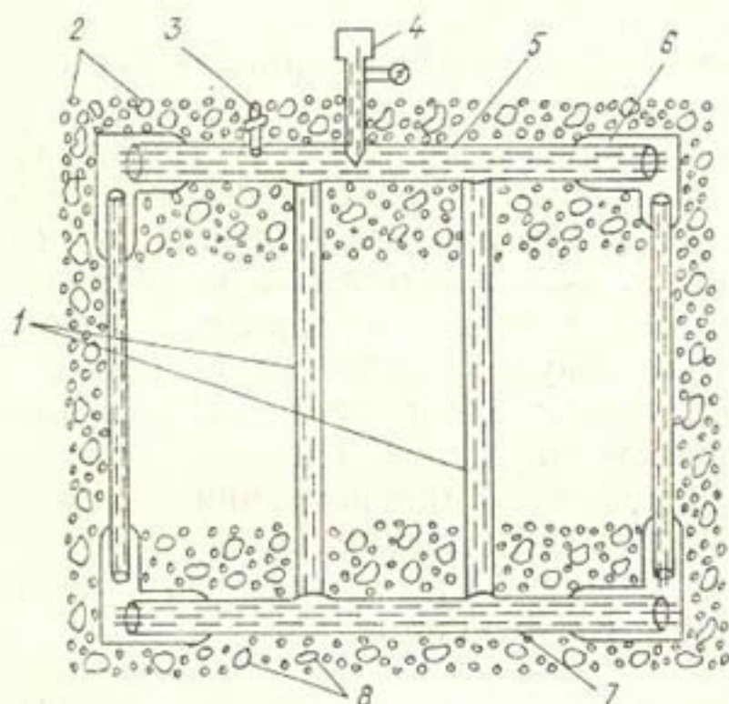
Рис. 6.4. Схема системы (устройства) полива сельскохозяйственных культур грунтовыми водами. 1 — непористые трубы, 2 — корнеобитаемый слой почвы, 3 — вентиль, 4 — тензиометр, 5 — пористая труба-увлажнитель, 6 — соединительная муфта, 7 — нижняя пористая труба, 8 — слой почвы, в котором залегают грунтовые воды.
