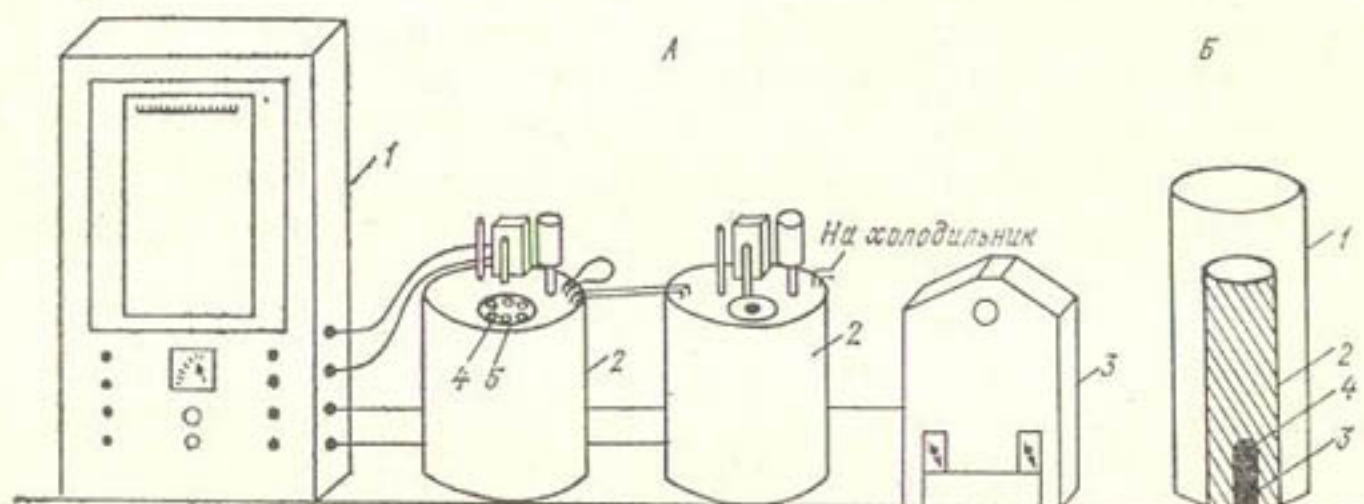
Рис. 2.11. Схема термопарного микропсихрометра.
