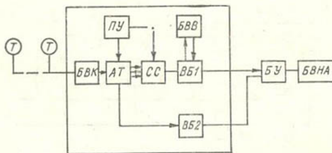
Рис. 6.2. Схема блока контроля состояния тензиометров.
