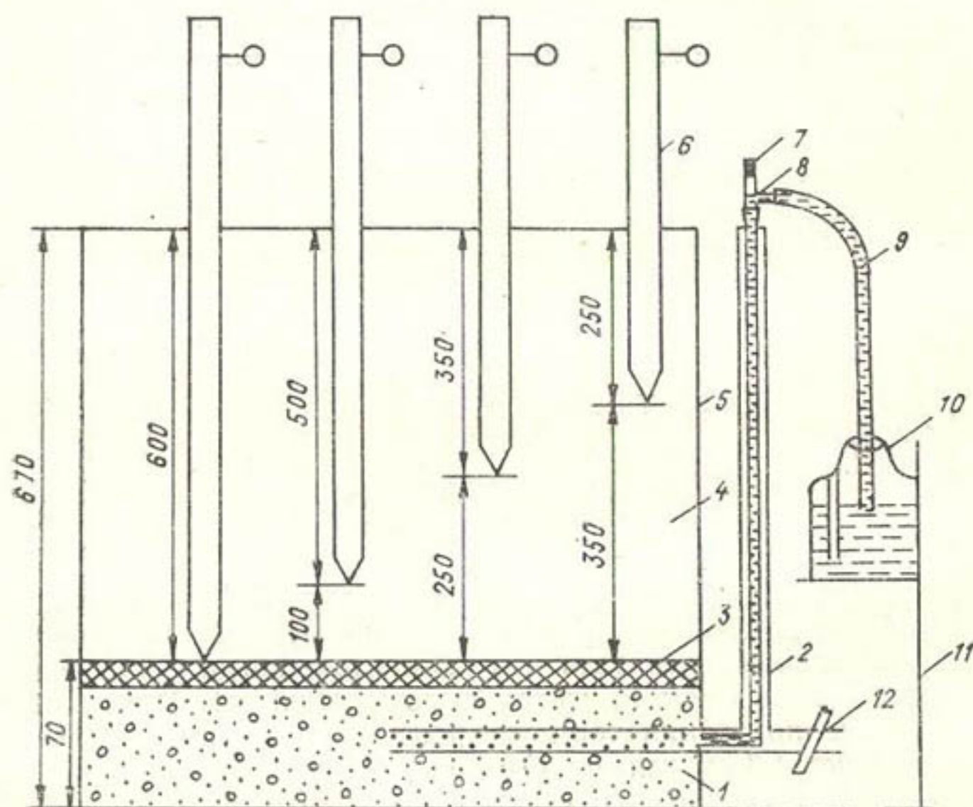
Рис. 2.9. Схема устройства для изучения капиллярных явлений почвенной влаги.
