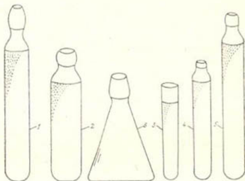
Рис. 2.3. Пористые керамические фильтры (датчики тензиометров) различной формы.
