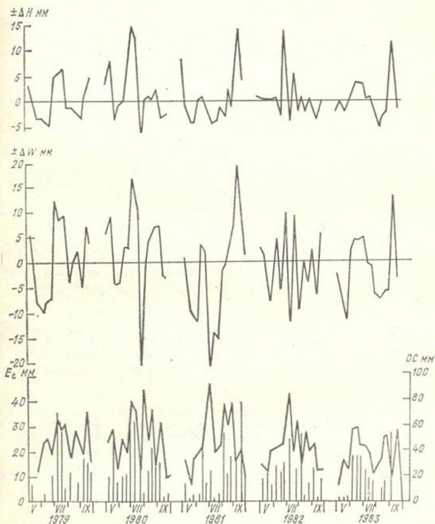
Рис. 4.9. Аккумуляция и расход влаги в ЗА ( \pm \Delta W ) и ГВ ( \pm \Delta H ) в аллювиальной луговой почве.
