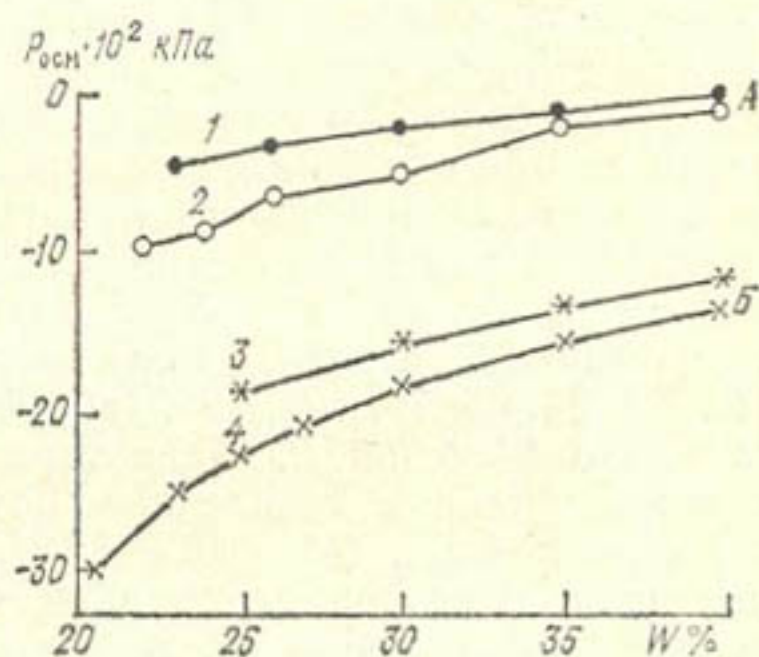
Рис. 3.11. Зависимость осмотического потенциала влаги P_{осм} от влажности в светло-каштановой почве (А) и солончаковом солонце (Б).
