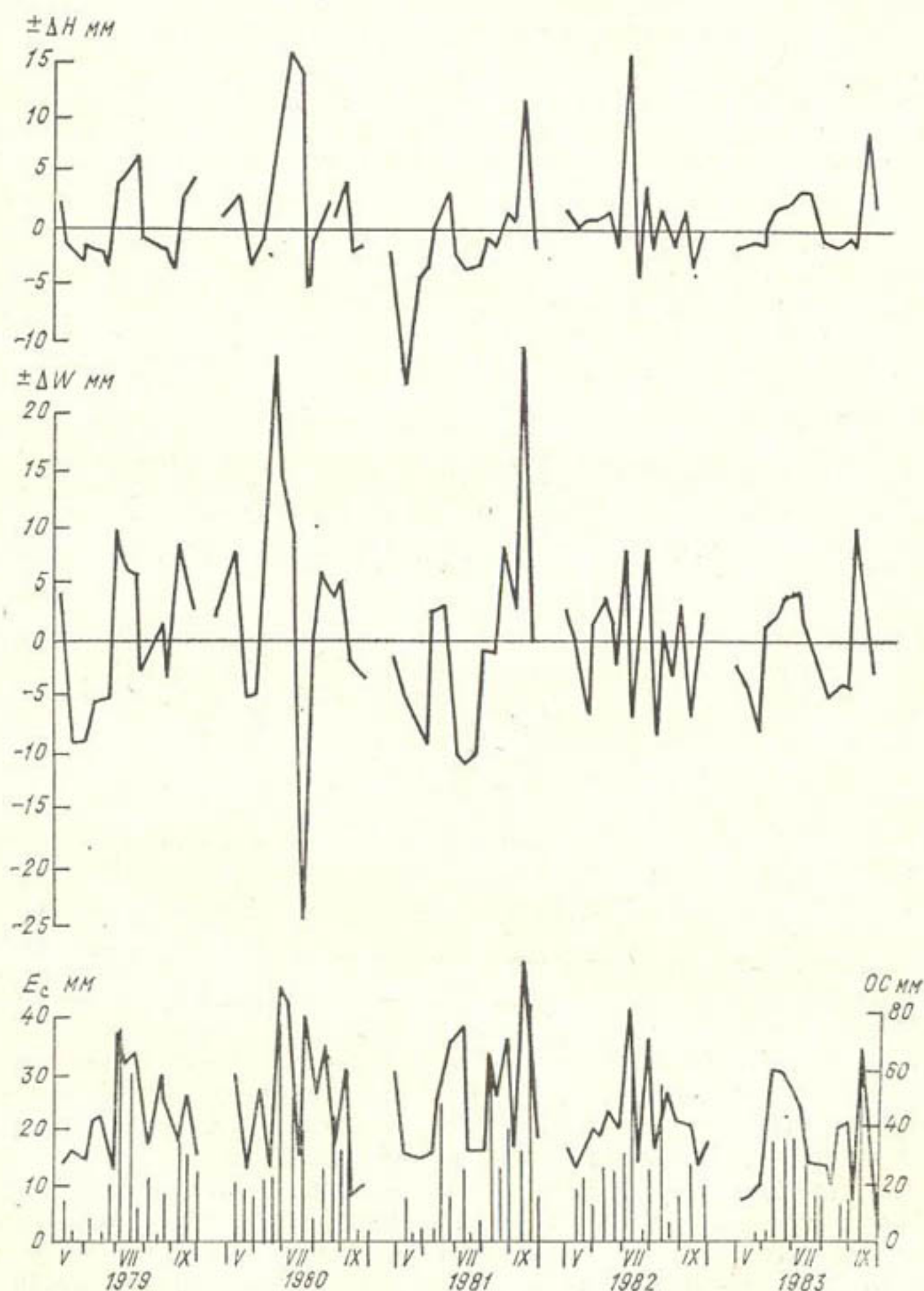
Рис. 4.8. Аккумуляция и расход влаги в ЗА ( \pm \Delta W ) и ГВ ( \pm \Delta H ) в дерново-подзолистой почве.
