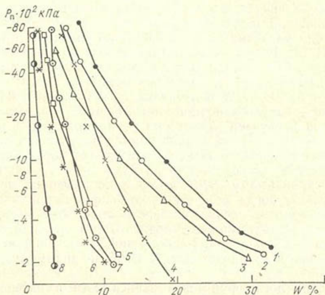
Рис. 3.2. Зависимость полного потенциала почвенной влаги P_{\Pi} от влажности почвы W , полученная психрометрическим методом.
