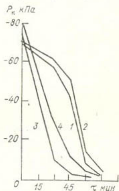
Рис. 2.2. Динамика потенциала влаги ( P_k ) в моно- лите дерново-подзолистой супесчаной почвы, поме- щенной в условия интенсивного испарения (Москов- ская обл.).
