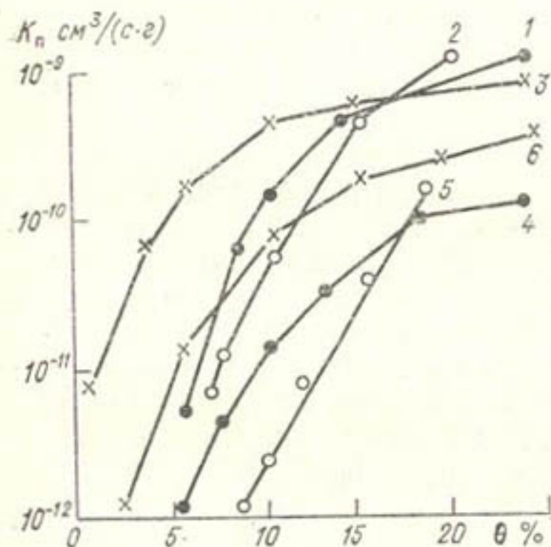
Рис. 4.3. Зависимость коэффициента влагопроводности K_n от объемной влажности \theta в черноземовидной супесчаной почве.
