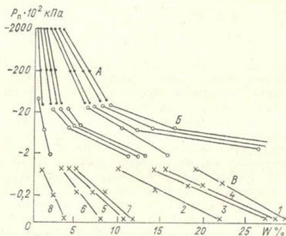
Рис. 3.3. Зависимость потенциала почвенной влаги от влажности почвы.
