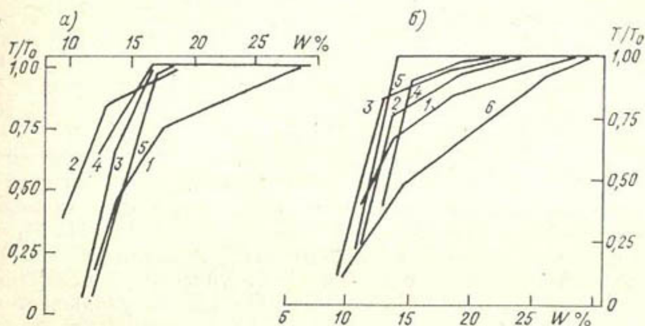
Рис. 5.9. Зависимость относительной транспирации ( T/T_0 ) овса от влажности пойменной черноземовидной суглинистой почвы.
