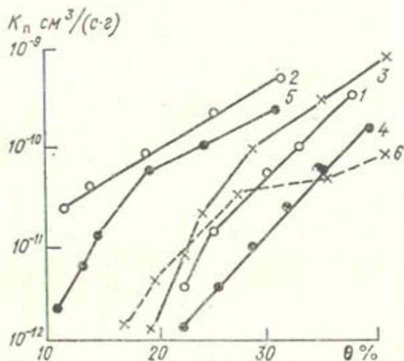
Рис. 4.4. Зависимость коэффициента влагопроводности K_n от объемной влажности \theta в пойменной черноземовидной суглинистой почве.
