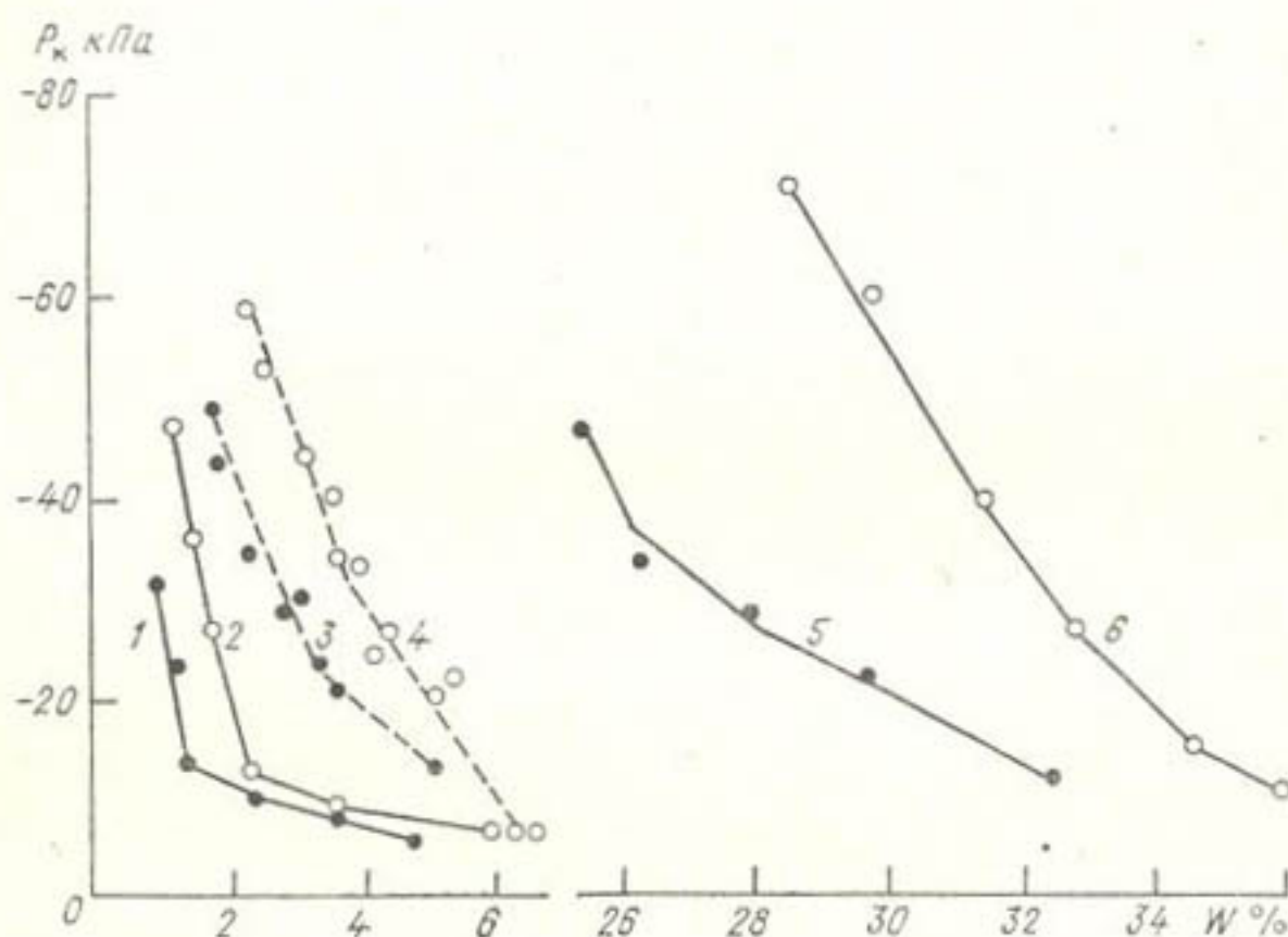
Рис. 3.14. Зависимость потенциала почвенной влаги P_k от влажности дерново-степной песчаной (1, 2), черноземовидной супесчаной (3, 4) и черноземовидной суглинистой (5, 6) почв при различной потенциальной транспирации: 11,5 мм водного слоя в сутки (1, 3, 5) и 3,5 мм водного слоя в сутки (2, 4, 6).
