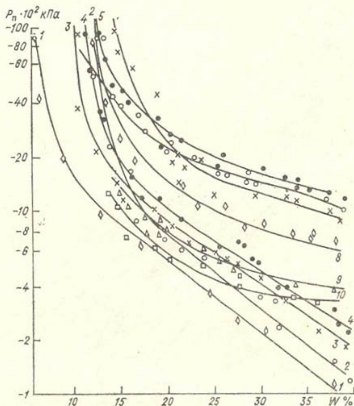
Рис. 3.8. Зависимость полного потенциала почвенной влаги P_{II} от влажности в светло-каштановой почве.
