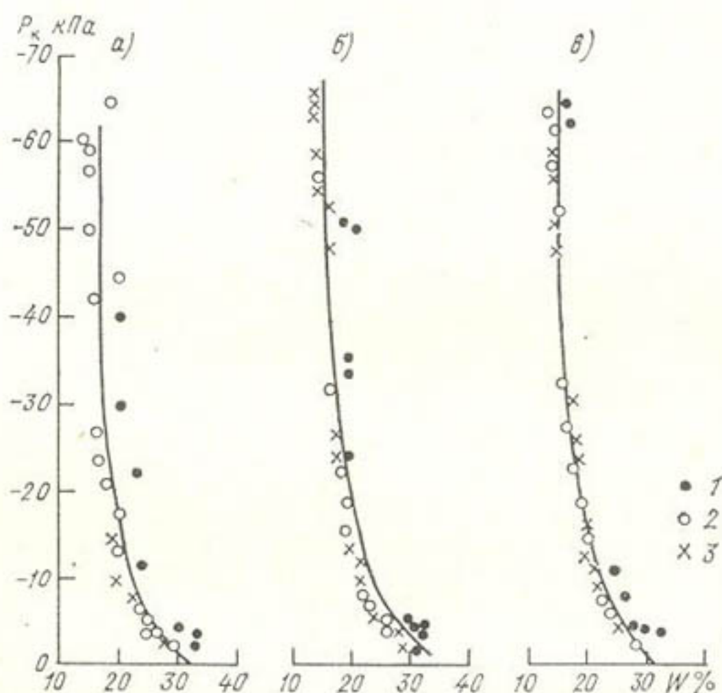
Рис. 3.16. Зависимость потенциала почвенной влаги P_k от влажности в мелиорированном солончаковом солонце Араратской равнины Армении (образцы ненарушенного сложения).
