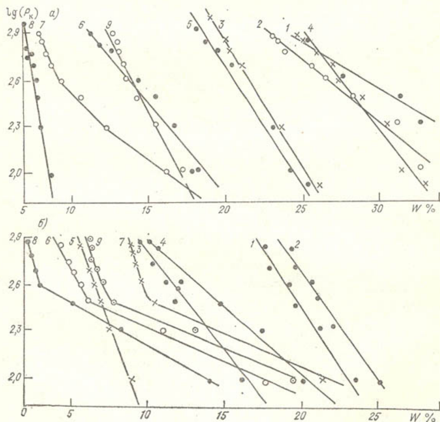
Рис. 3.1. Зависимость капиллярно-сорбционного потенциала почвенной влаги ново-подзолистой Слой почвы: 1) 10—20 см, 2) 20—30 см, 3) 45—55 см, 4) 70—80 см, 5) 95—105 см, 6) 120—
