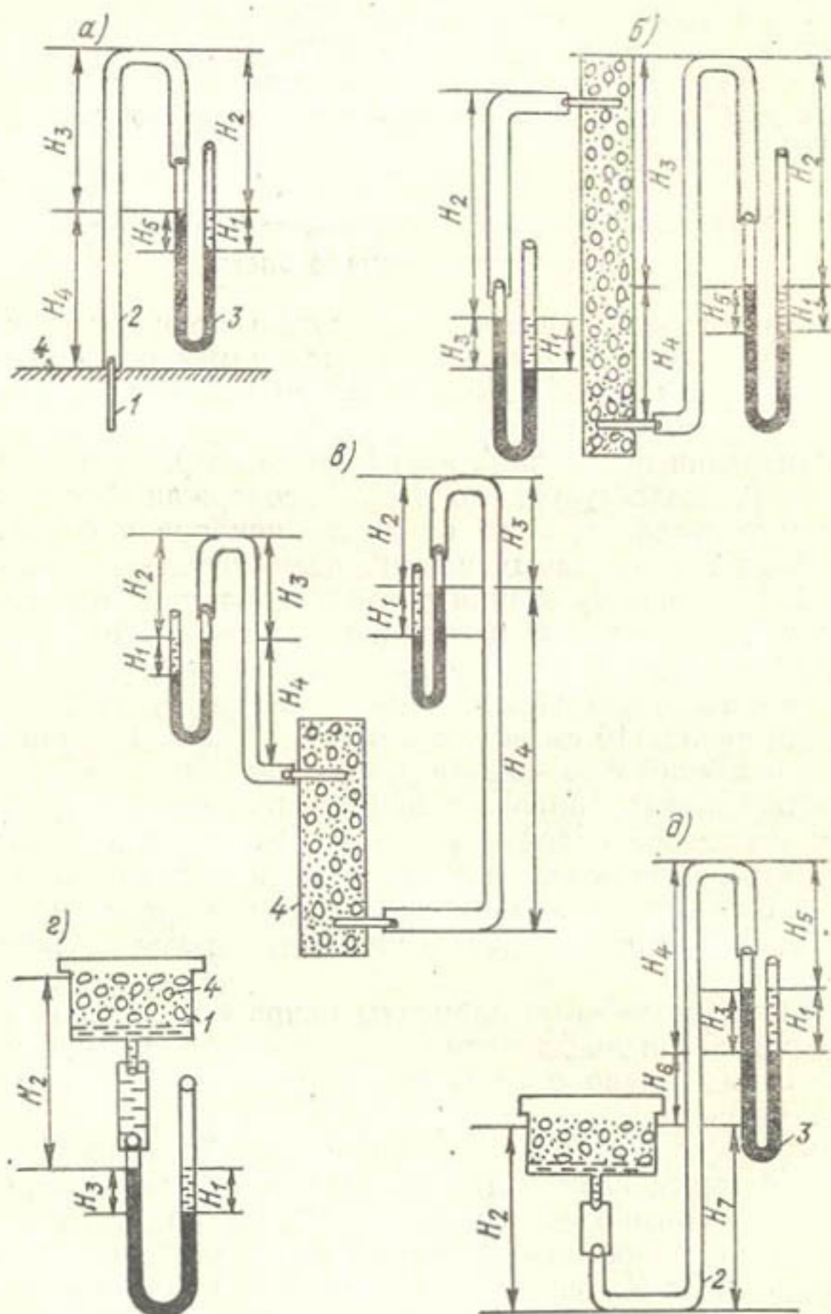
Рис. 2.6. Схемы расположения основных частей тензиометров (а—в) и капилляриметров (г, д) для обоснования поправок к их показаниям.
