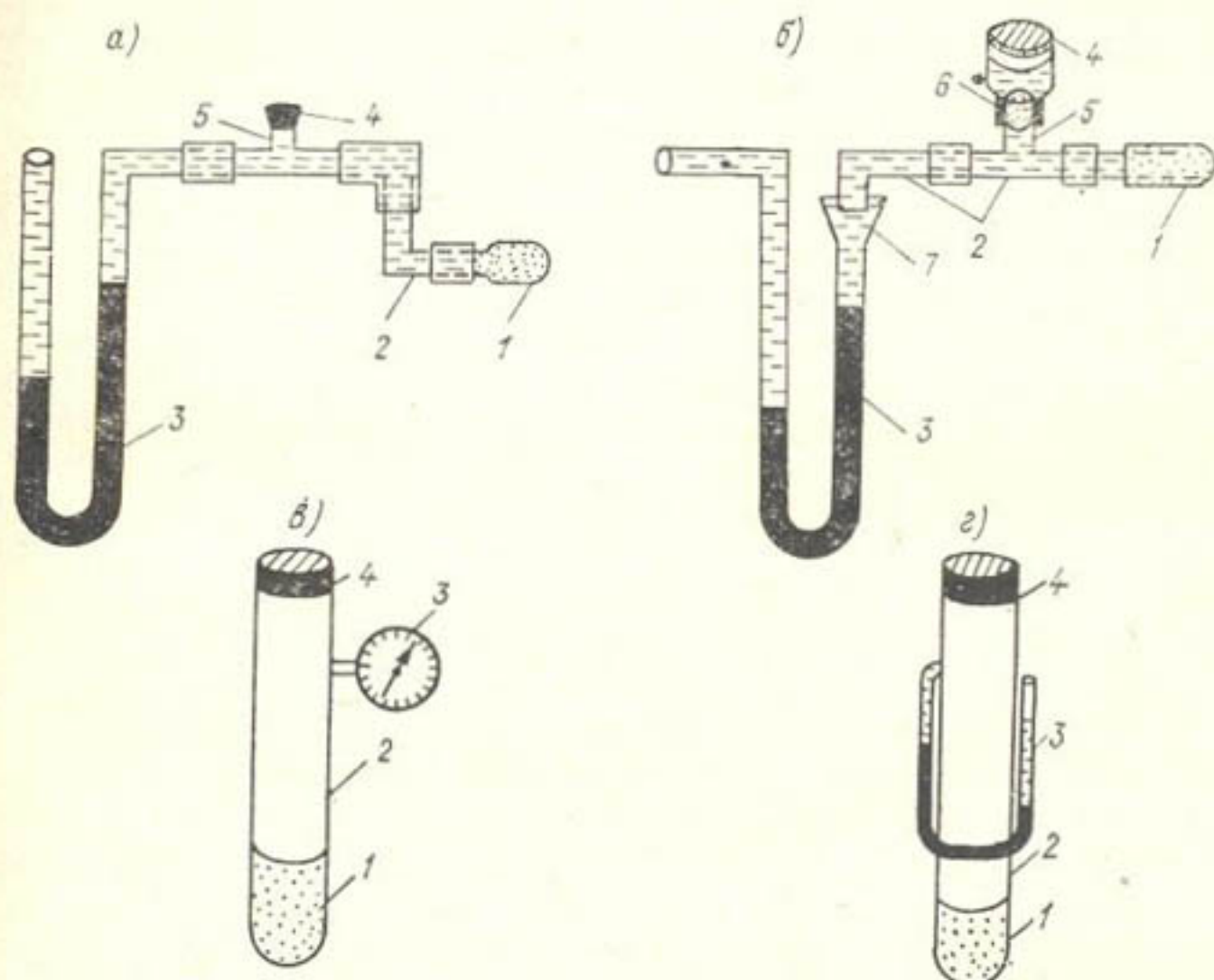
Рис. 2.1. Схемы тензиометров.
