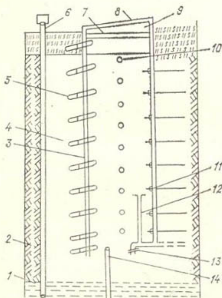
Рис. 2.4. Схема армированного почвенного разреза для установки тензиометров.
