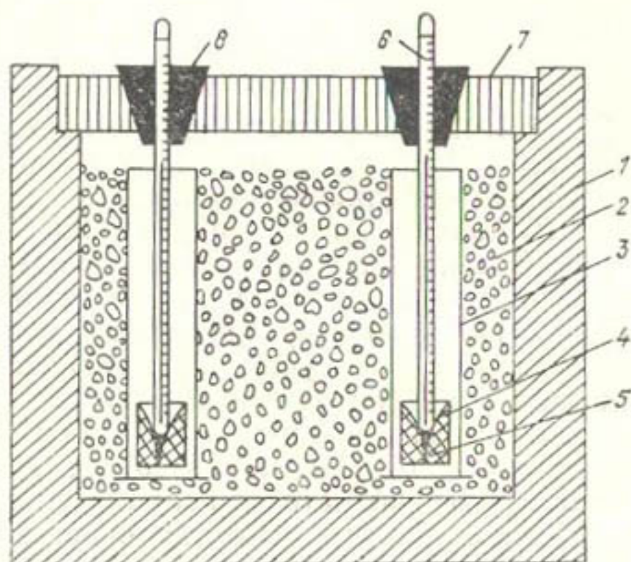
Рис. 2.10. Схема криоскопа.
