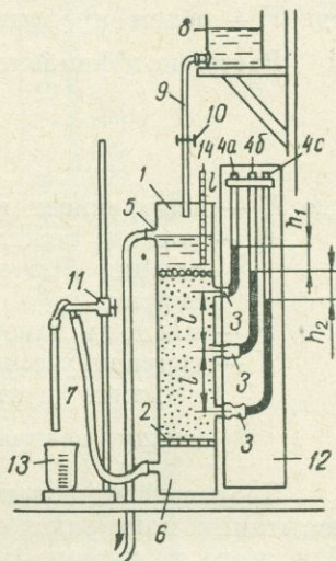
Рис. IV-4. Прибор Тима.
