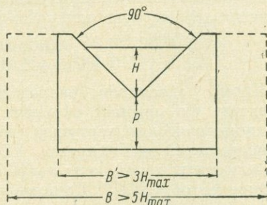
Рис. XII-15. Водослив Томсона.
