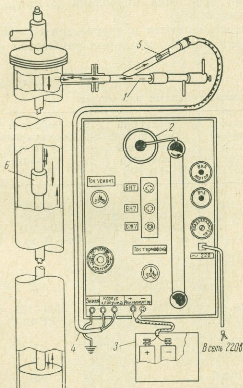
Рис. XII-31. Эхолот ЭС-50.
