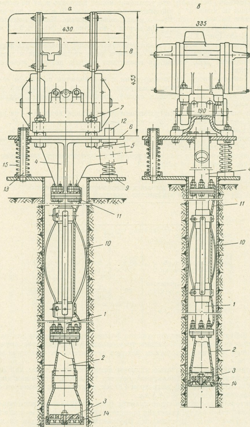
Рис. XI-3. Вибрационный водоподъемник.
