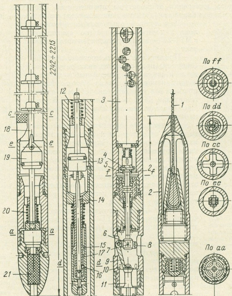
1 — проводок; 2 — клетка; 3 — часовой механизм; 4 — фрикцион; 5 — вал; 6 — гайка; 7 — штифт; 8 — кольцо; 9 — палец; 10 — переходный патрубков; 11 — крестовина; 12 — пружина; 13 — верхний клапан; 14 — игла; 15 — корпус; 16 — шарик; 17 — колпак; 18 — шток; 19 — нижний клапан; 20 — пружина; 21 — хвостовик.
