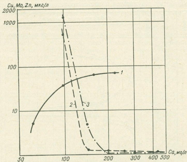
Рис. VI-4. Зависимость содержаний микроэлементов от содержаний кальций-иона в грунтово-трещинных водах Алматы.
