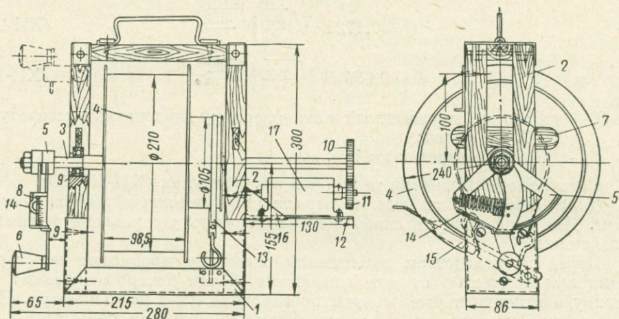
Рис. XII-29. Аппарат Яковлева легкого типа.
