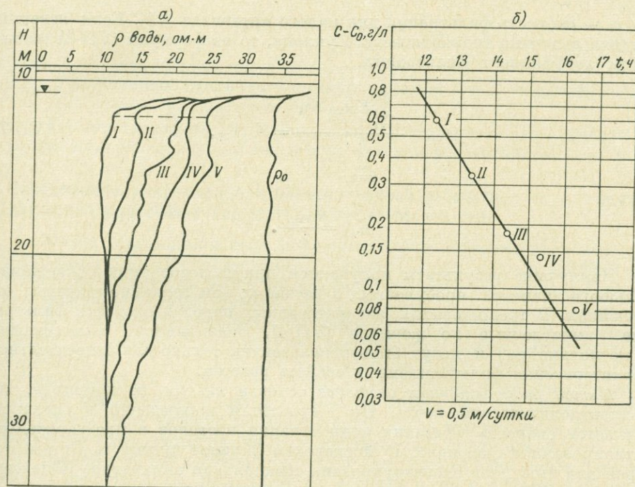
Рис. VII-5. Пример обработки результатов наблюдений электролитическим методом.
