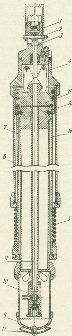
Рис. XII-20. Телеско- пический пробоотборник Е. В. Симонова.
