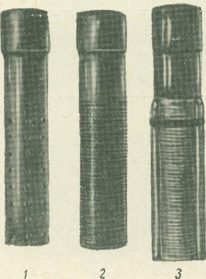
Рис. X-5. Обмотка тканей из стекловолокна на каркас фильтра.
