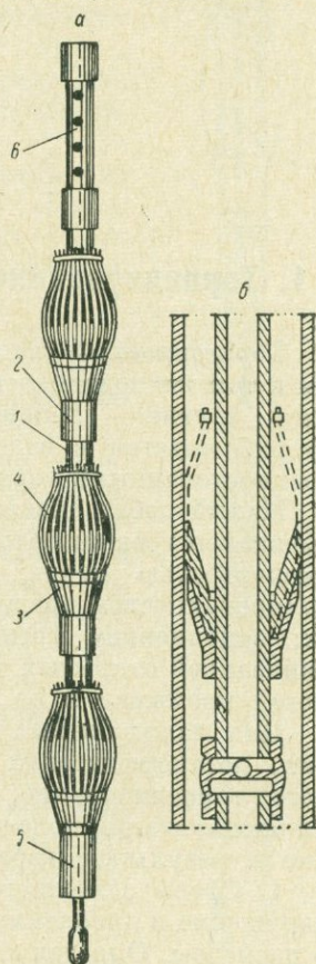
Рис. XII-41. Сваб. a — внешний вид поршня; б — деталь корзинки и обратного шарового клапана поршня;
