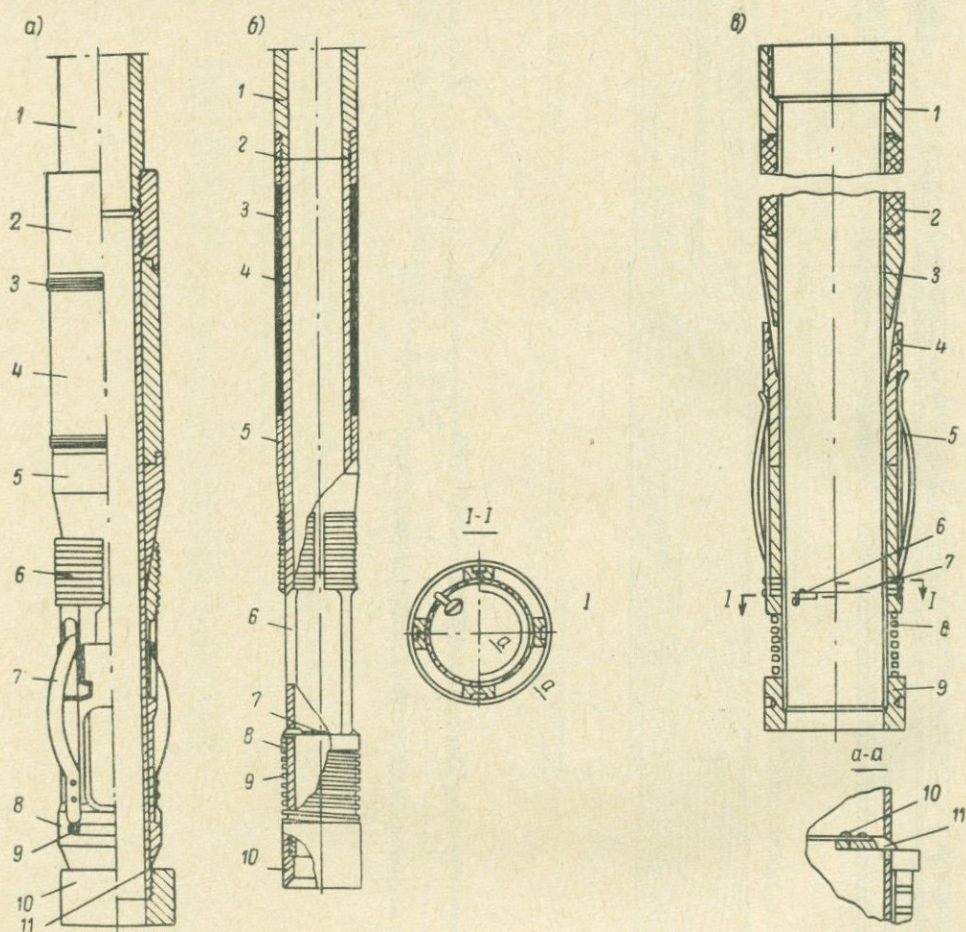
Рис. XIV-9. Стенные пакеры.
