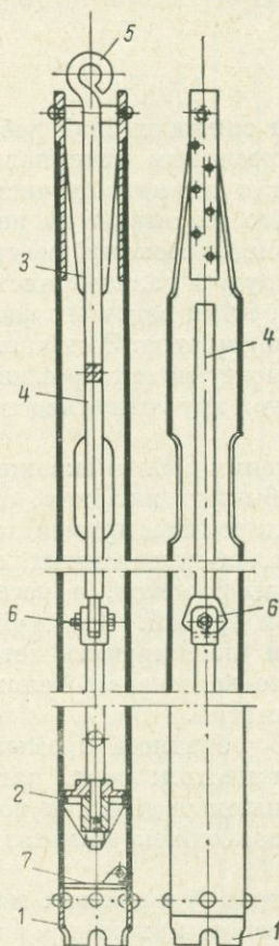
Рис. XIII-8. Поршневая колонка.
