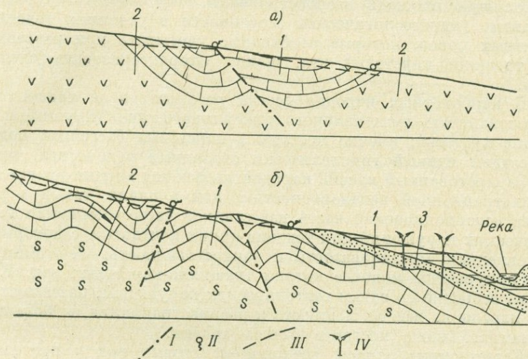
Рис. VIII-2. Месторождения трещинно-карстовых вод (второй тип). а — замкнутый бассейн с фронтом потока трещинно-карстовых вод до 3—5 км и мощностью горизонта 150—300 м; б — открытый бассейн трещинно-карстовых вод значительной площади распространения, мощность горизонта — 300—1000 м.
