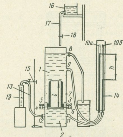
Рис. IV-6. Прибор Г. Н. Каменского.
