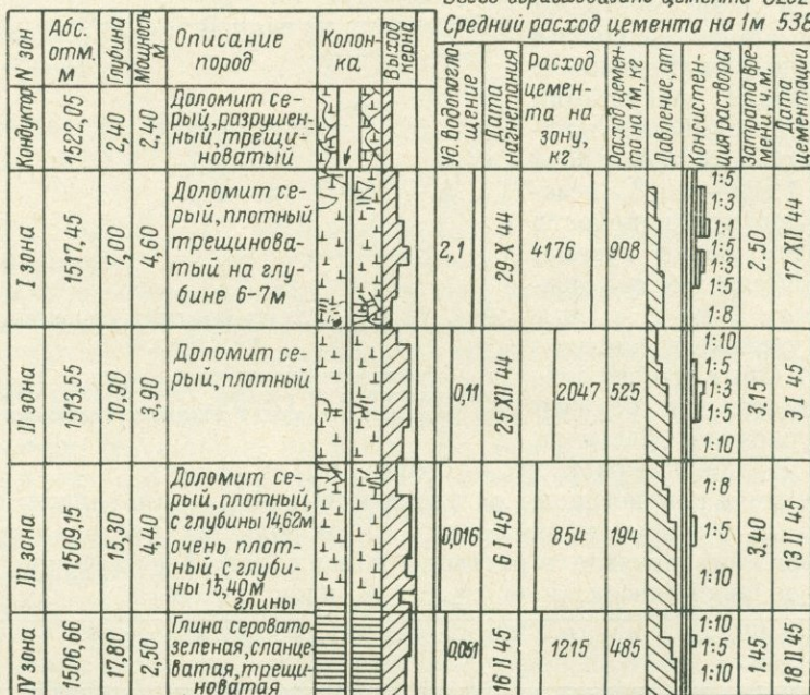
Всего зацементировано 15,4 м Всего израсходовано цемента 8292 кг Средний расход цемента на 1 м 538 кг
